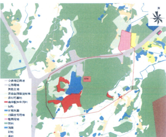
用地规划图
