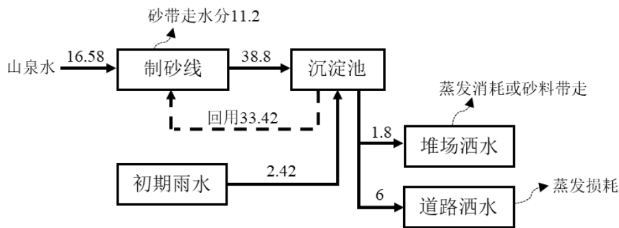
图7 水平衡示意图(单位m 3 /d)
