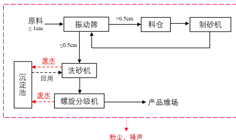
图6 制砂线工艺流程图
